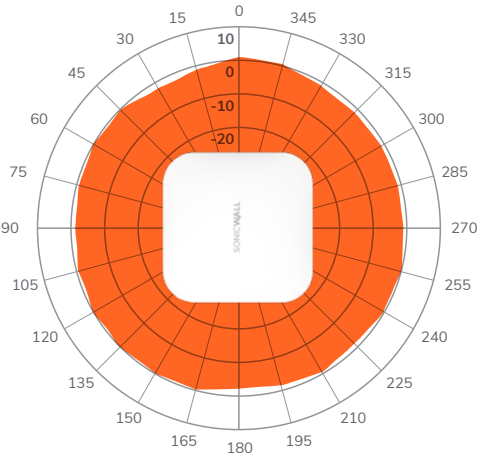
2.4GHz, YZ-Plane
