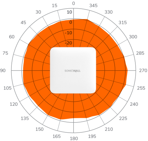
5GHz, XY-Plane
