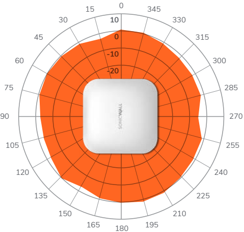
5GHz, YZ-Plane
