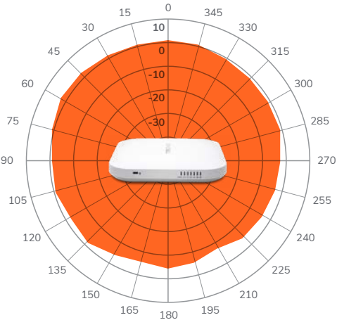
5GHz, XZ-Plane
